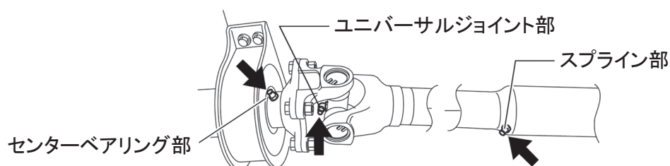
《大型トラック給脂箇所（例）》
