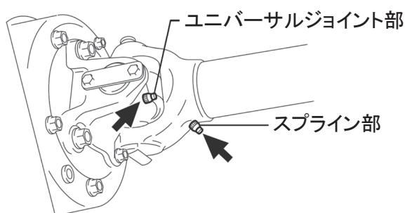
《大型バス給脂箇所（例）》
