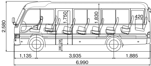
BDG-XZB50M GX (諸元表番号③)
