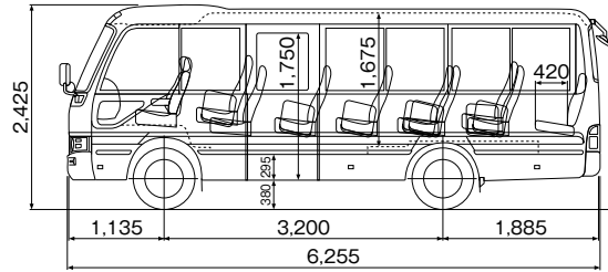
PDG-XZB40M LX (諸元表番号④)
