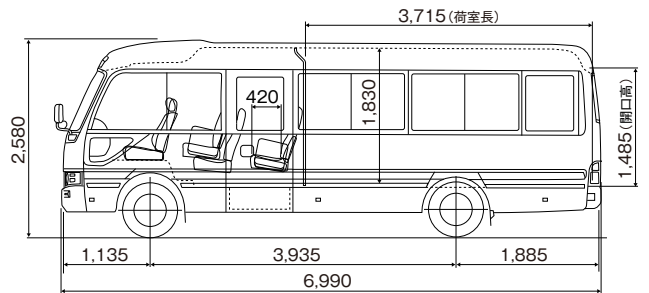
PDG-XZB56Y BIG VAN (諸元表番号⑥)
