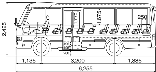
PDG-XZB40M 幼児専用車 (諸元表番号⑤)
