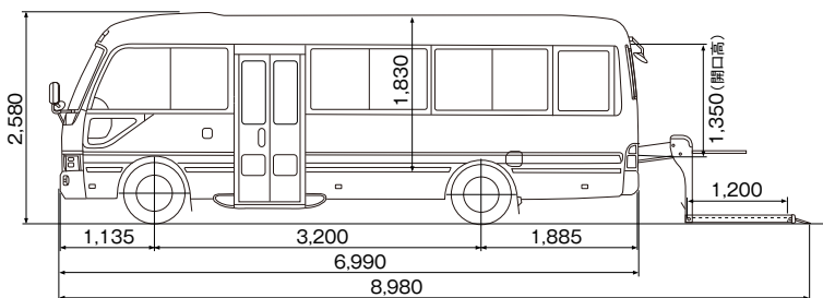
PDG-XZB50M リフトサービスバス LX (諸元表番号⑦)
