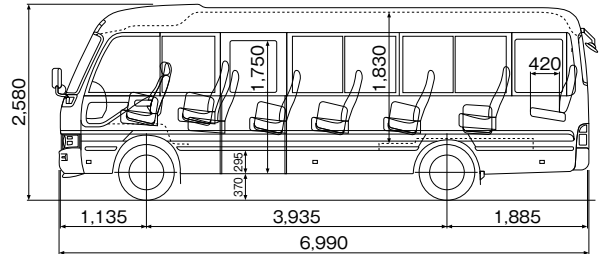
BDG-XZB51M EX (諸元表番号②)
