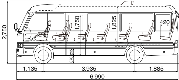
BDG-XZB51M スーパーラウンジ (諸元表番号①)
