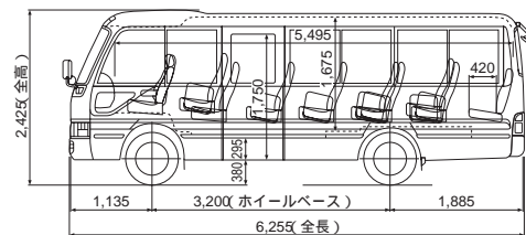
LX4WD (BB) ロングボデー ハイルーフ 29人乗り
