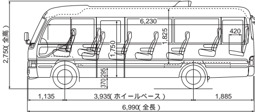
スーパーラウンジ (HDB) ロングボデー ハイルーフ 20人乗り
