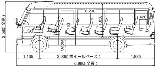
LX (HZB) ロングボデー ハイルーフ 29人乗り
