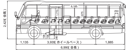
幼児専用車 (HZB) ロングボデー 標準ルーフ 大人3人 + 幼児49人乗り
