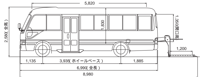
リフトサービスバス (HZB) ロングボデー ハイルーフ 22人 + 車いす2人乗り
