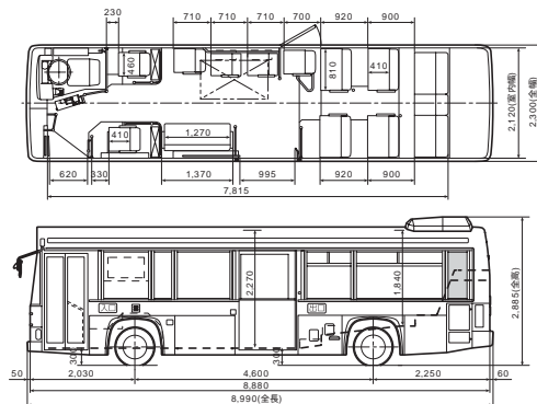
乗合(路線)ノンステップ(9m車) HR1JKEE 単区間(前乗・中降)都市型
