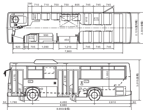
乗合(路線)ノンステップ(9m車) HR1JKEE 単区間(前乗・中降)都市型
