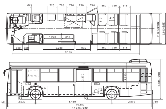
乗合(路線)ノンステップ(10.5m車) HR1JNEE 単区間(前乗・中降)都市型
